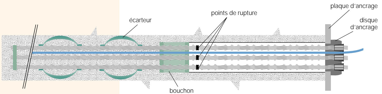
Tirant câble démontable
