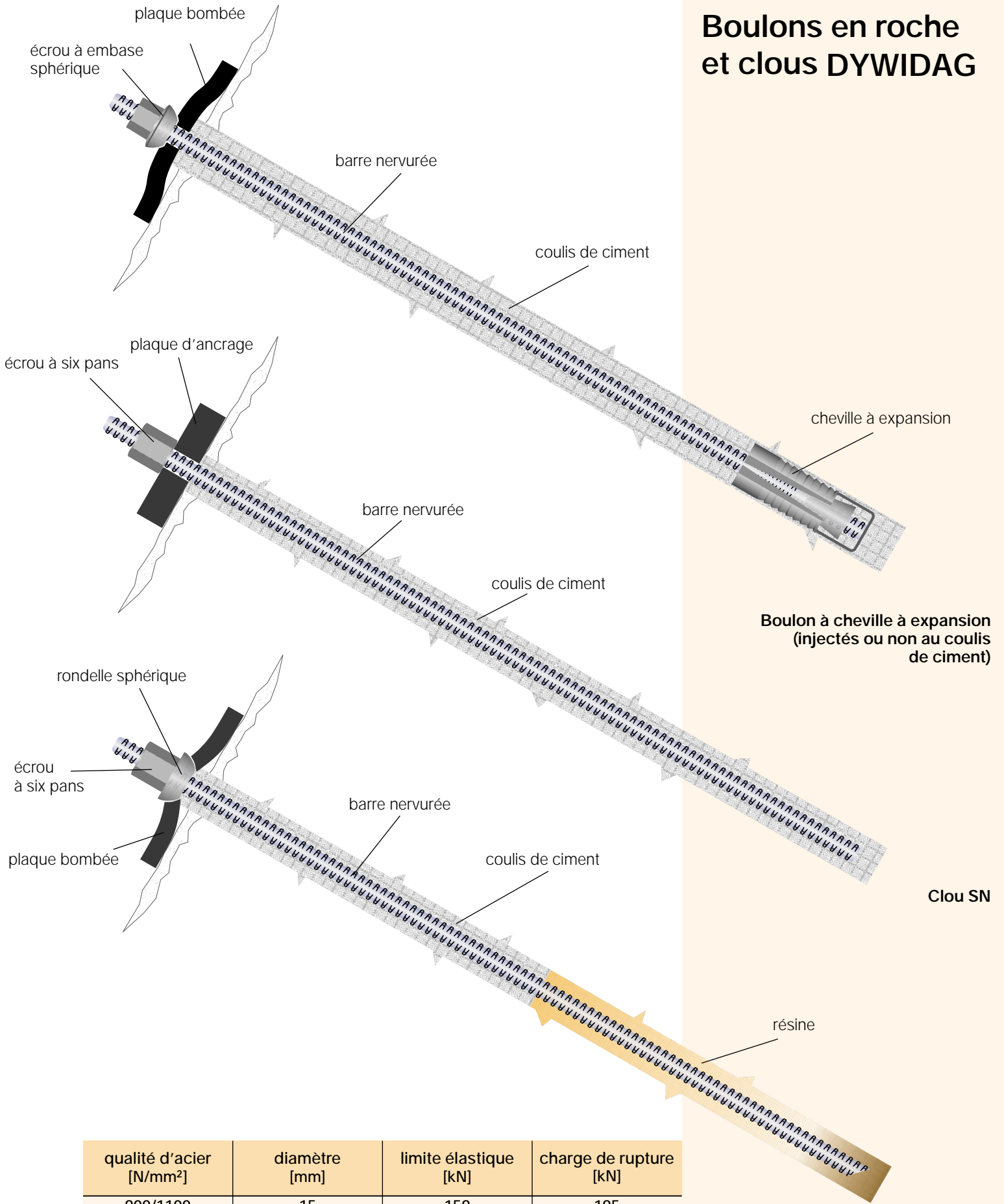
Boulon à la résine
