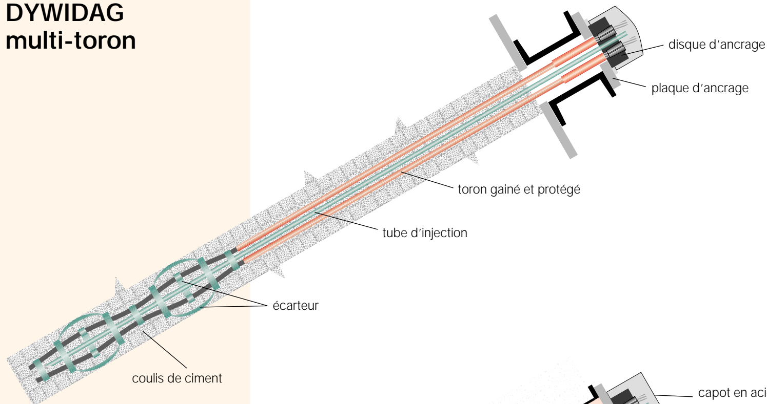
Tirant provisoire
